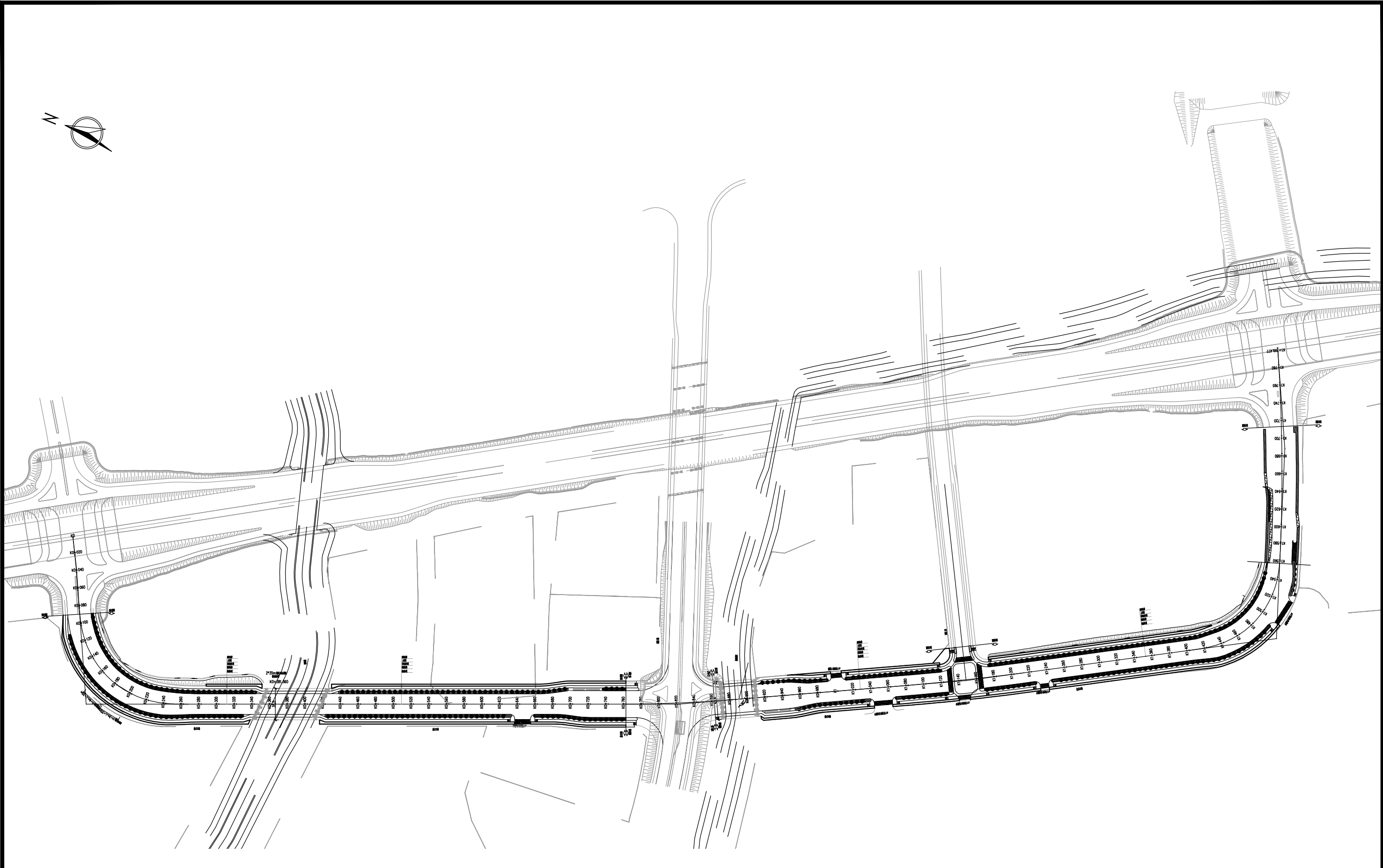
知识城技术五路市政道路及配套工程绿化总平面图 1:4000
